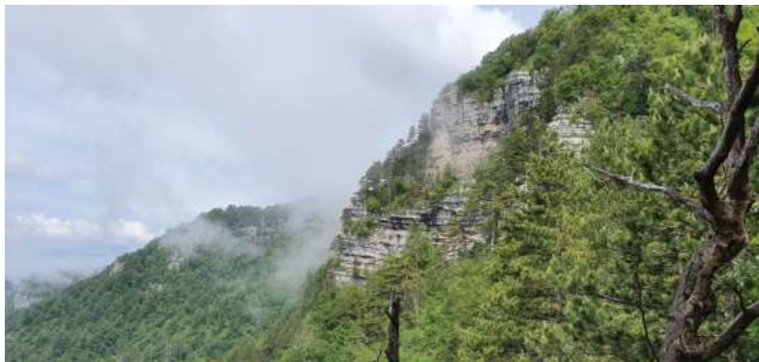
Slika 3: Prepadne stene kanjona Kolpe pod Krokarjem
