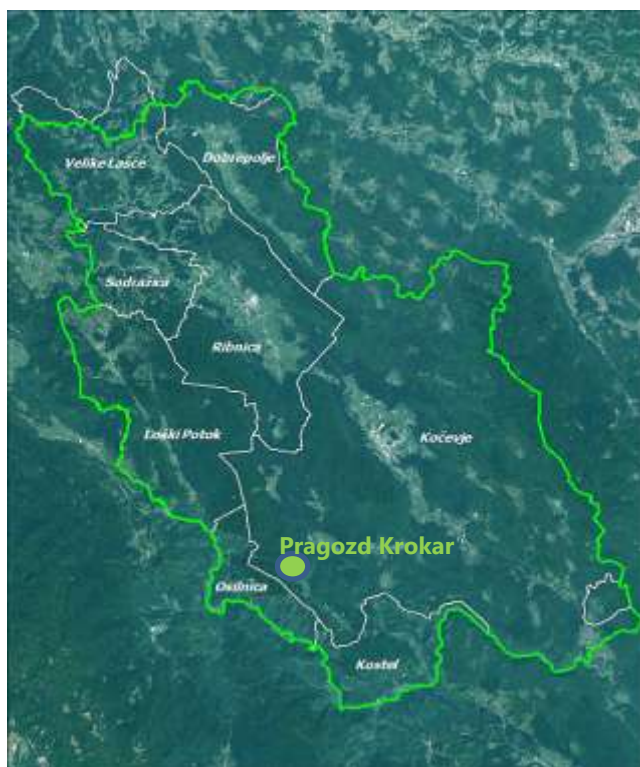
Slika 4, 5: Makro in mikro lokacija GR Pragozda Krokara
